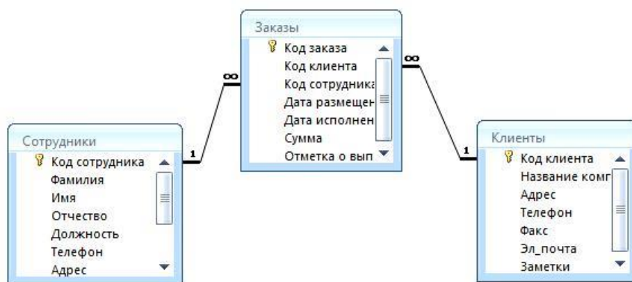
Рис. 2. Схема данных
