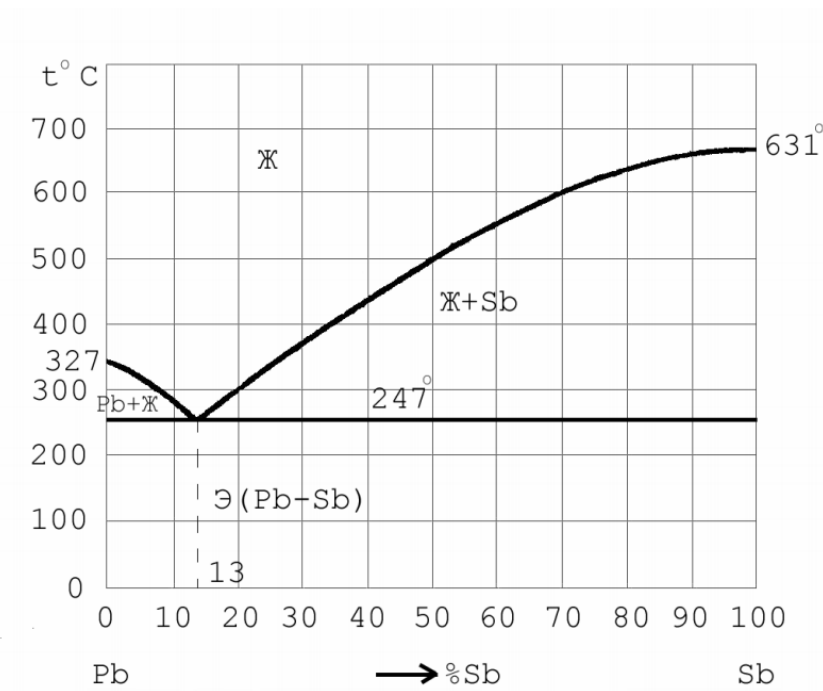
Рис.9. Диаграмма состояния системы Pb – Sb
