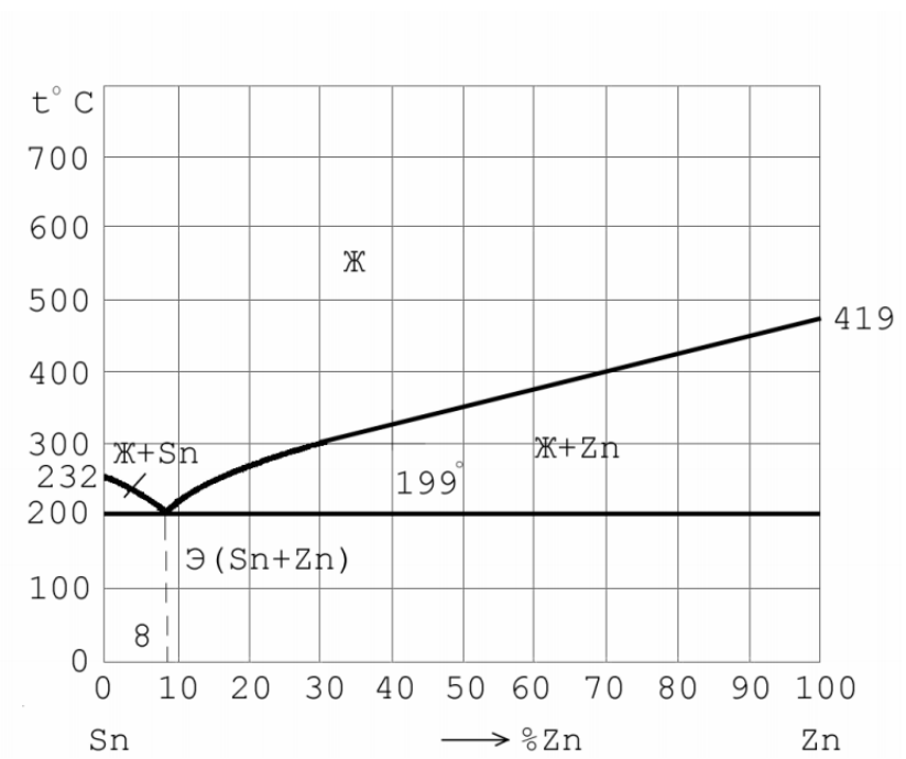
Рис.10. Диаграмма состояния системы Sn – Zn
