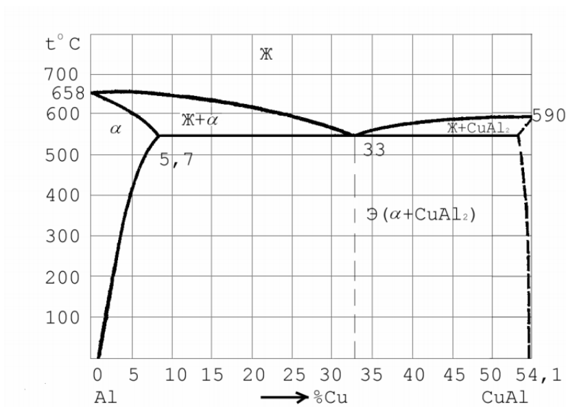
Рис.8. Диаграмма состояния системы Al – CuAl 2
