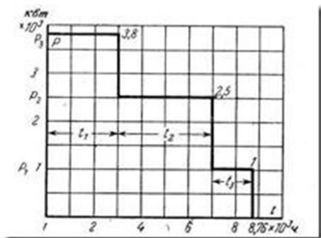
Рисунок 1 - Ступенчатый график нагрузки предприятия
