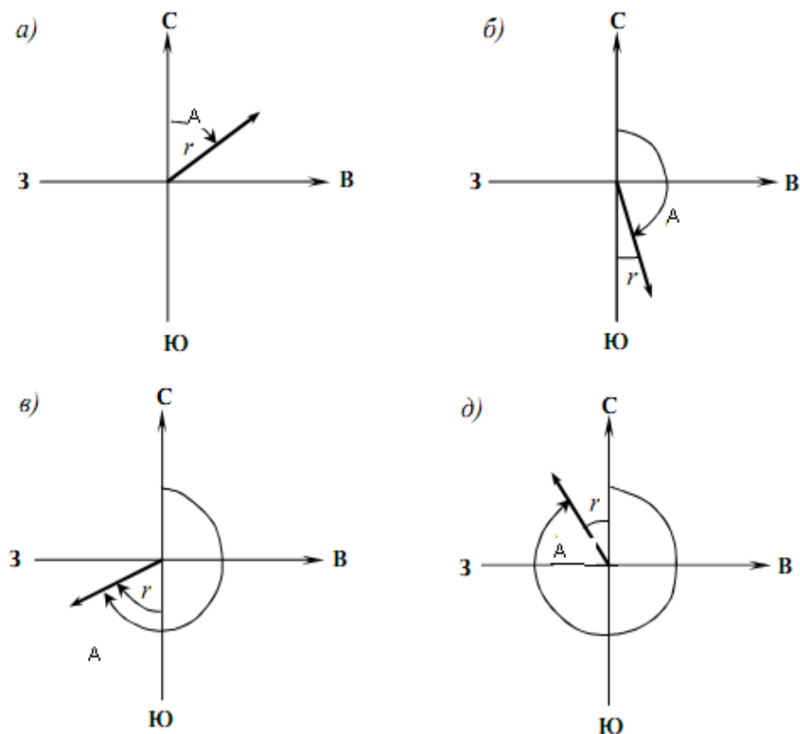
Рисунок 7 – Румбы направлений
