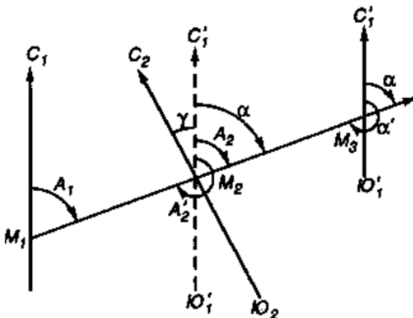
Рисунок 8. Определение дирекционного угла
