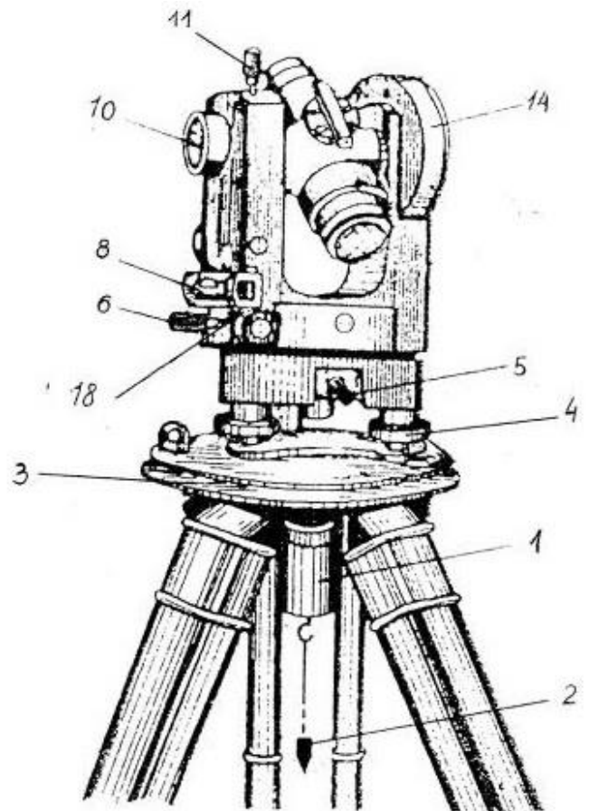
Теодолит 2Т30
