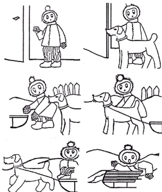
Рис. 6. Последовательность событий
