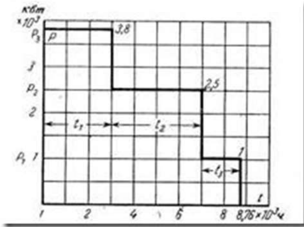
Рисунок 1 - Ступенчатый график нагрузки предприятия
