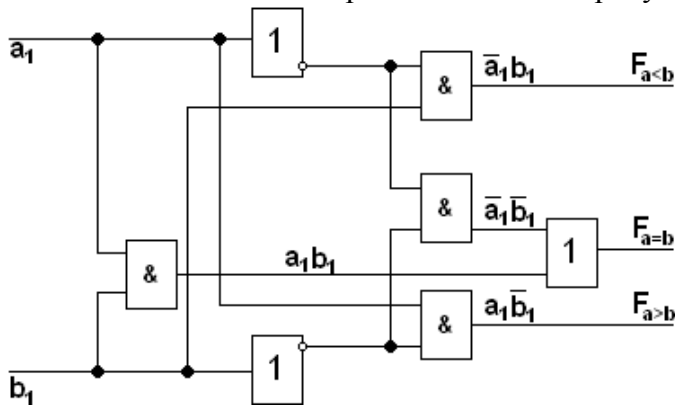
(а) Одноразрядный компаратор
