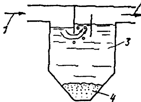
Рис. 1. Схема ротоклона
