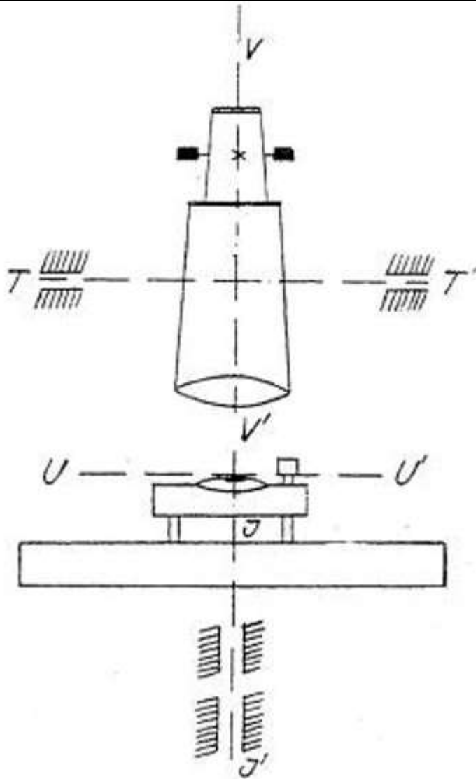
Рис. Схема осей теодолита
