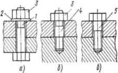
Рис. 64. Резьбовые соединения: а — болтовое, б — шпильчное, в — винтовое, 1 — болт, 2 — шайба, 3 — гайка, 4 — шпилька, 5 — винт
