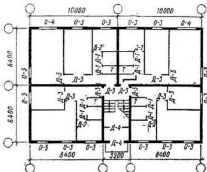
Графическая работа № 14 Построение планов здания
