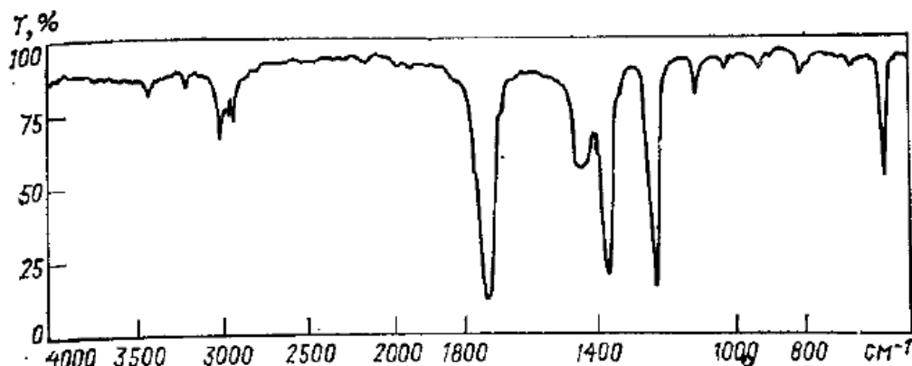
Рис. 1.8. ИК-спектр ацетона
