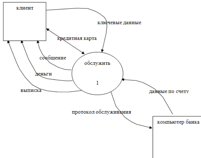
Рис. 2. Контекстная диаграмма банковской задачи
