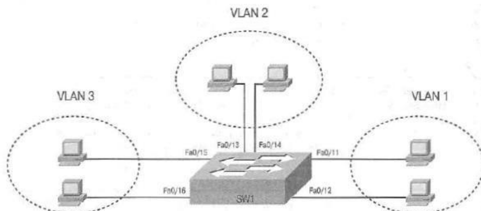
Рисунок 1 – Сеть с одним коммутатором и тремя VLAN-сетями
