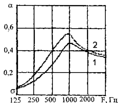
Рисунок 1.3 - Частотные характеристики коэффициента поглощения пористых материалов
