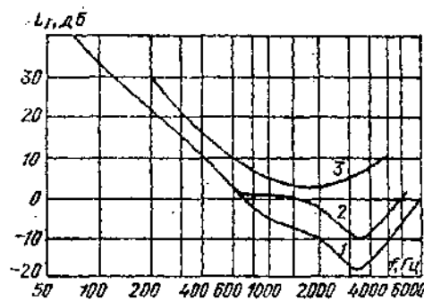
Рисунок 2.1 - Частотная зависимость уровней порога слышимости
