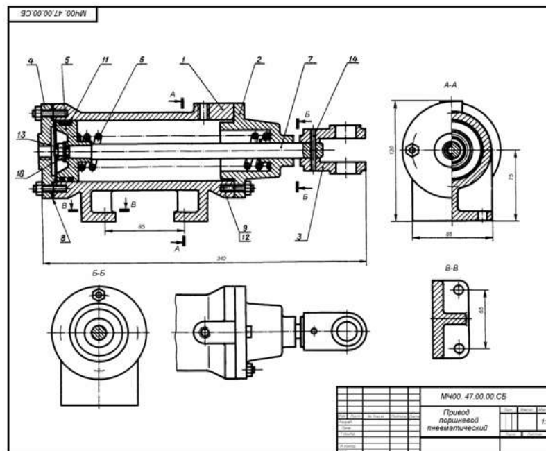
Графическая работа № 8. Сборочный чертеж;
