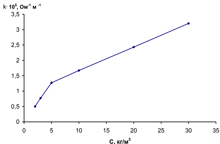
Рис. 9. Графическое определение ККМ раствора лаурата натрия Как следует из рисунка, ККМ равна 5 кг/м³.
