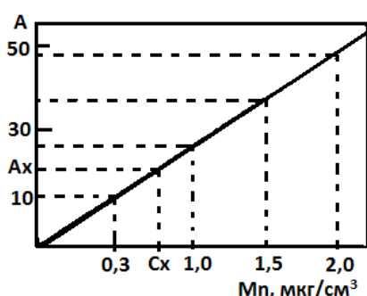
Рис. 3. Градуировочный график в координатах C_{ст} - A_{ст} .
