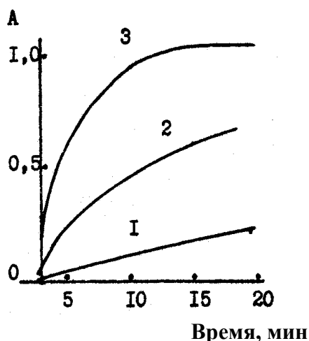
19. Рис. 1. I – 278, 2 – 295, 3 – 330 К. Исходные концентрации реагирующих компонентов равны 5 \cdot 10^{-3} моль/л. Протекает реакция \text{A} + \text{B} = \text{C} + \text{D}
