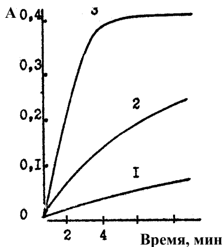
21. Рис. 3. I – 280, 2 – 290, 3 – 300 К. Концентрации A и B равны 2 \cdot 10^{-3} моль/л.
