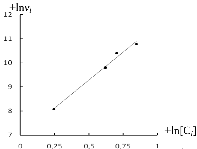
Рис.1. Графическое определение кинетических порядков сорбции ионов ТМ глиной при 295 К
