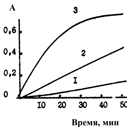
22. Рис. 4. I – 278, 2 – 288, 3 – 295 К. Концентрации A и B равны 1 \cdot 10^{-5} моль/л.
