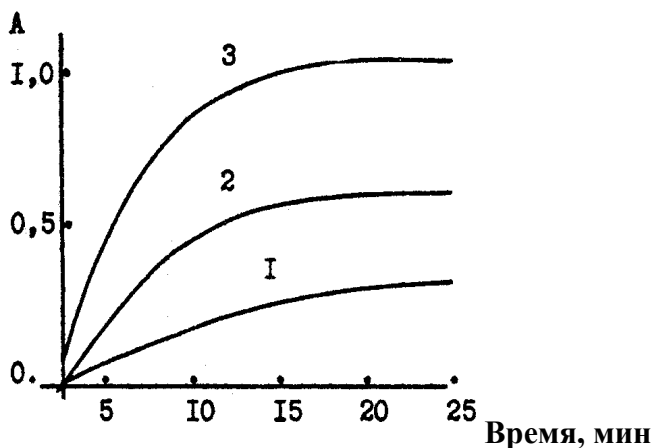
20. Рис. 2. I – 278, 2 – 295, 3 – 330 К. Исходные концентрации реагирующих компонентов равны 5 \cdot 10^{-3} моль/л. Протекает реакция \text{A} + \text{B} = \text{C} + \text{D}
