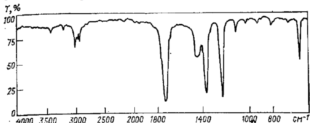
Рис. 1.8. ИК-спектр ацетона
