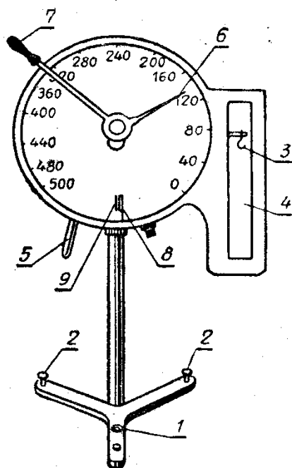
Рис. 5. Торзионные весы.
