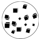
Рис.1. Кристаллы \text{K}_2\text{PbCu}(\text{NO}_2)_6
