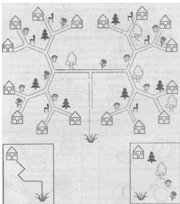
Рис. 5. Лабиринт
