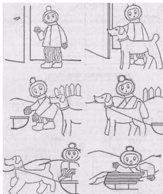
Рис. 6. Последовательность событий
